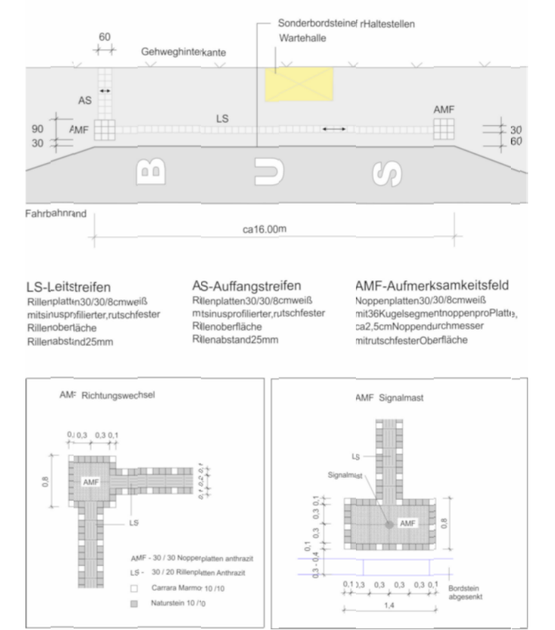
Prinzipskizze Haltestellen
