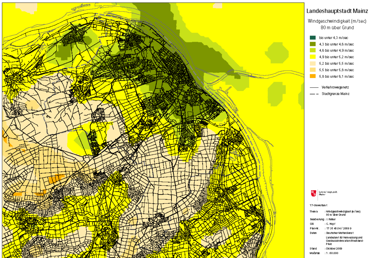
Abbildung 5: Karte der Windgeschwindigkeit im Stadtgebiet Mainz (unmaßstäblich)
