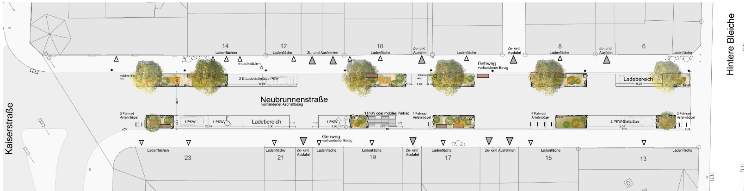
Grundriss (ohne Maßstab)
