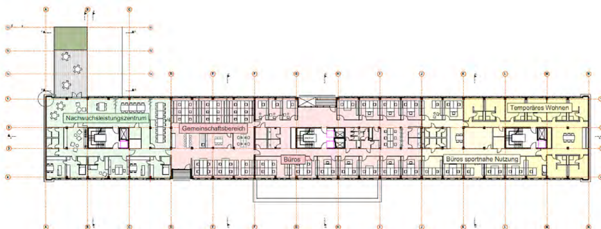
Abbildung 8 Entwurfsplanung 2. OG
