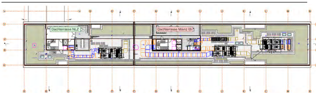
Abbildung 10 Entwurfsplanung DG, Dachaufsicht
