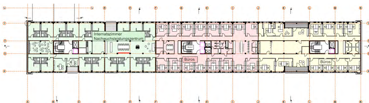
Abbildung 7 Entwurfsplanung 3. OG
