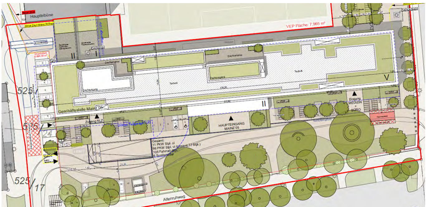
Abbildung 3 Ausschnitt aus dem Vorhaben- und Erschließungsplan Quelle: Faerber Architekten
