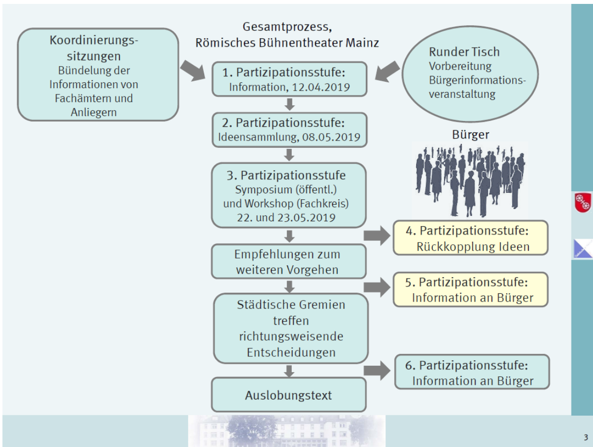
Ablaufschema Partizipation
