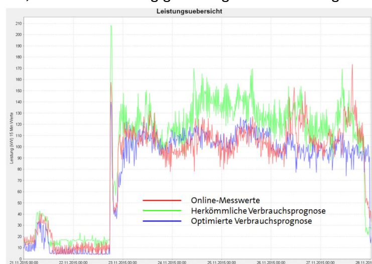
Abbildung 9: Online-Messwerte
