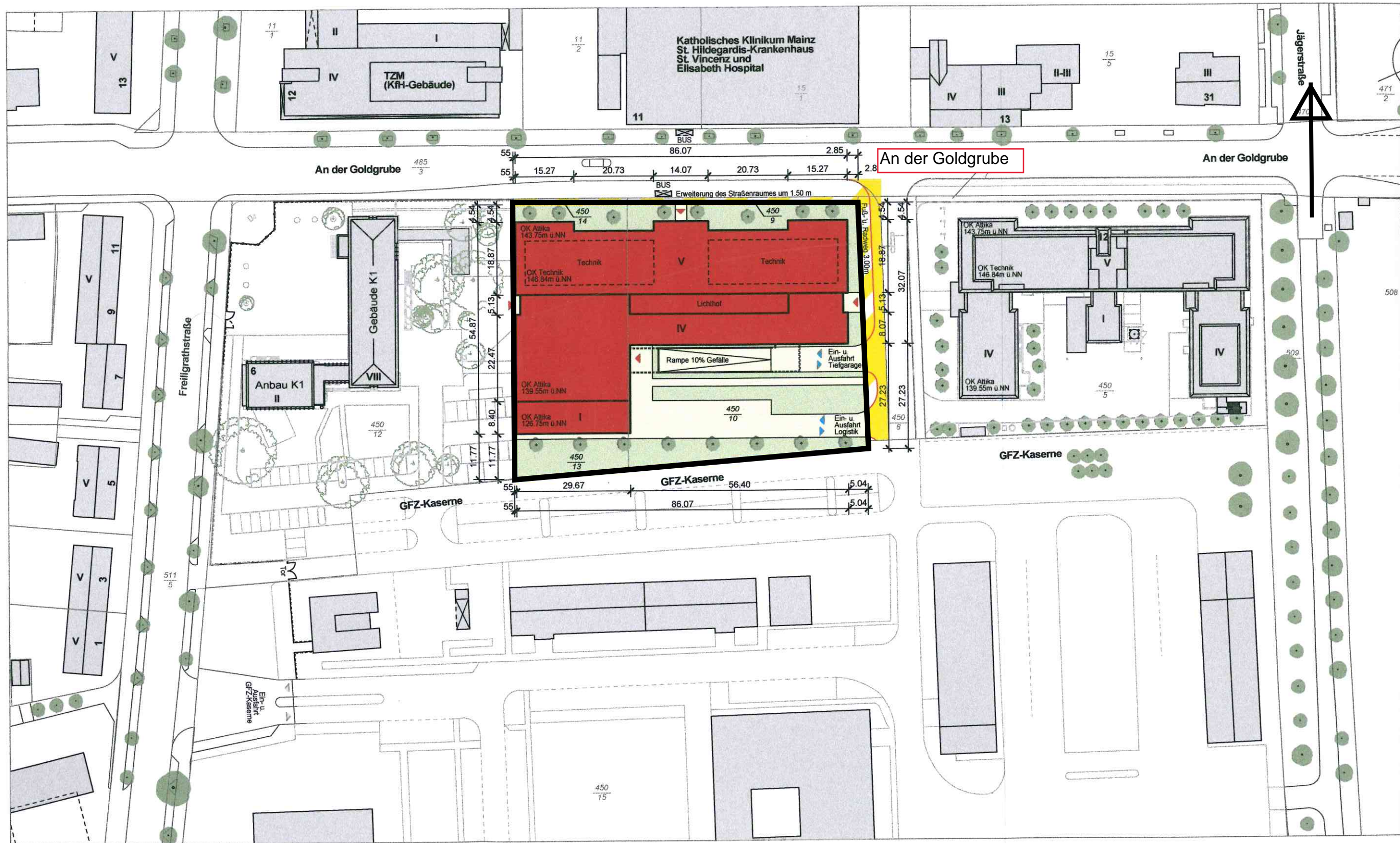
Lageplan, Maßstab 1:1000
