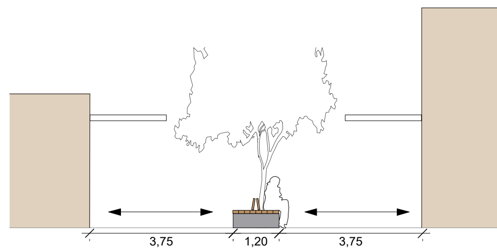
Ansicht | Doppelbank | 1:100
