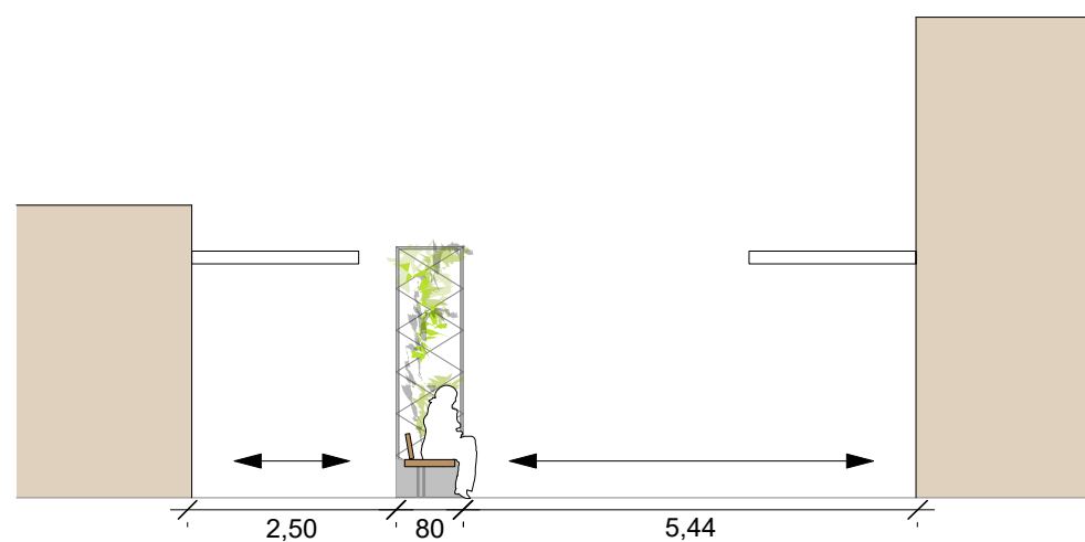
Ansicht | Bank mit Rankgerüst | 1:100
