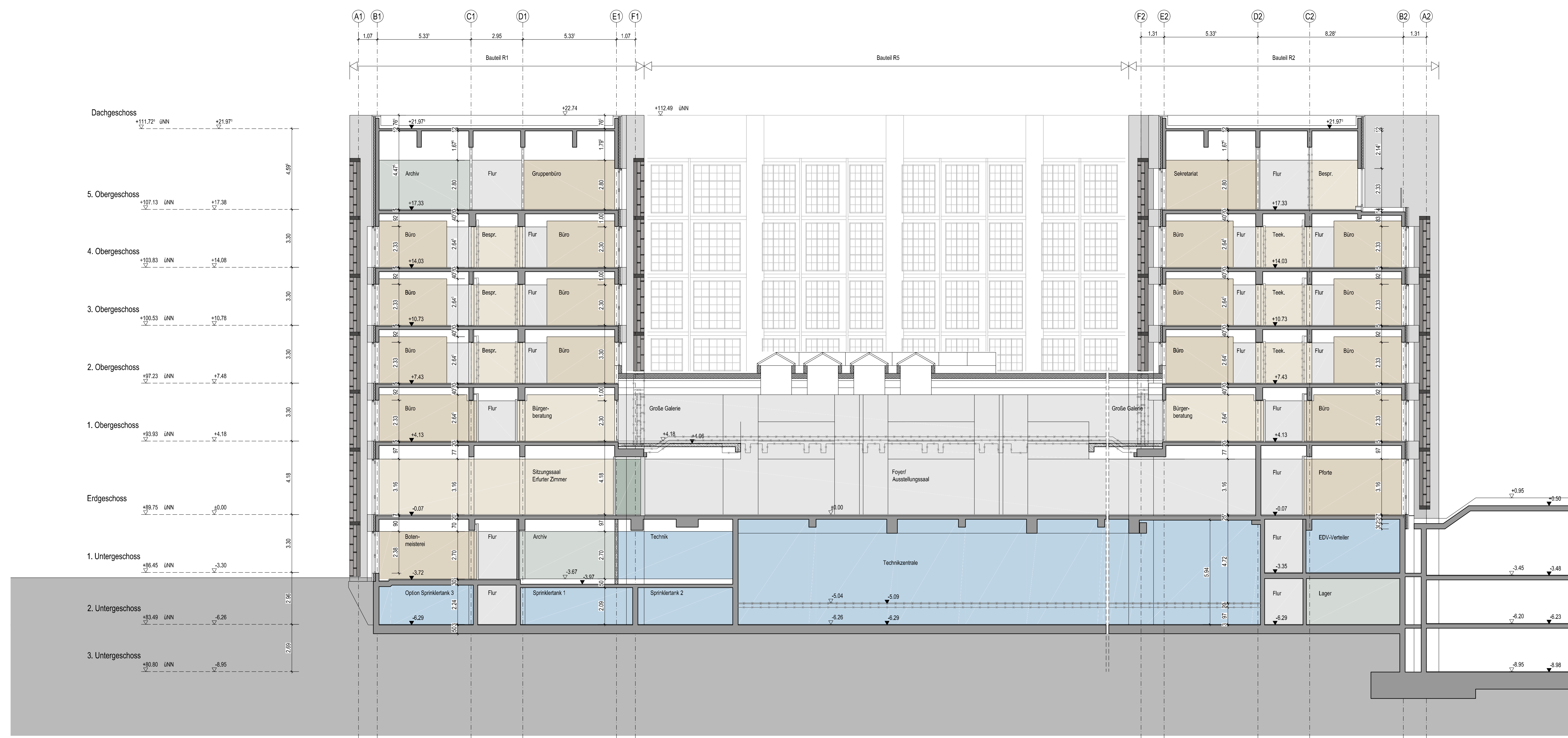
Schnitt B-B
