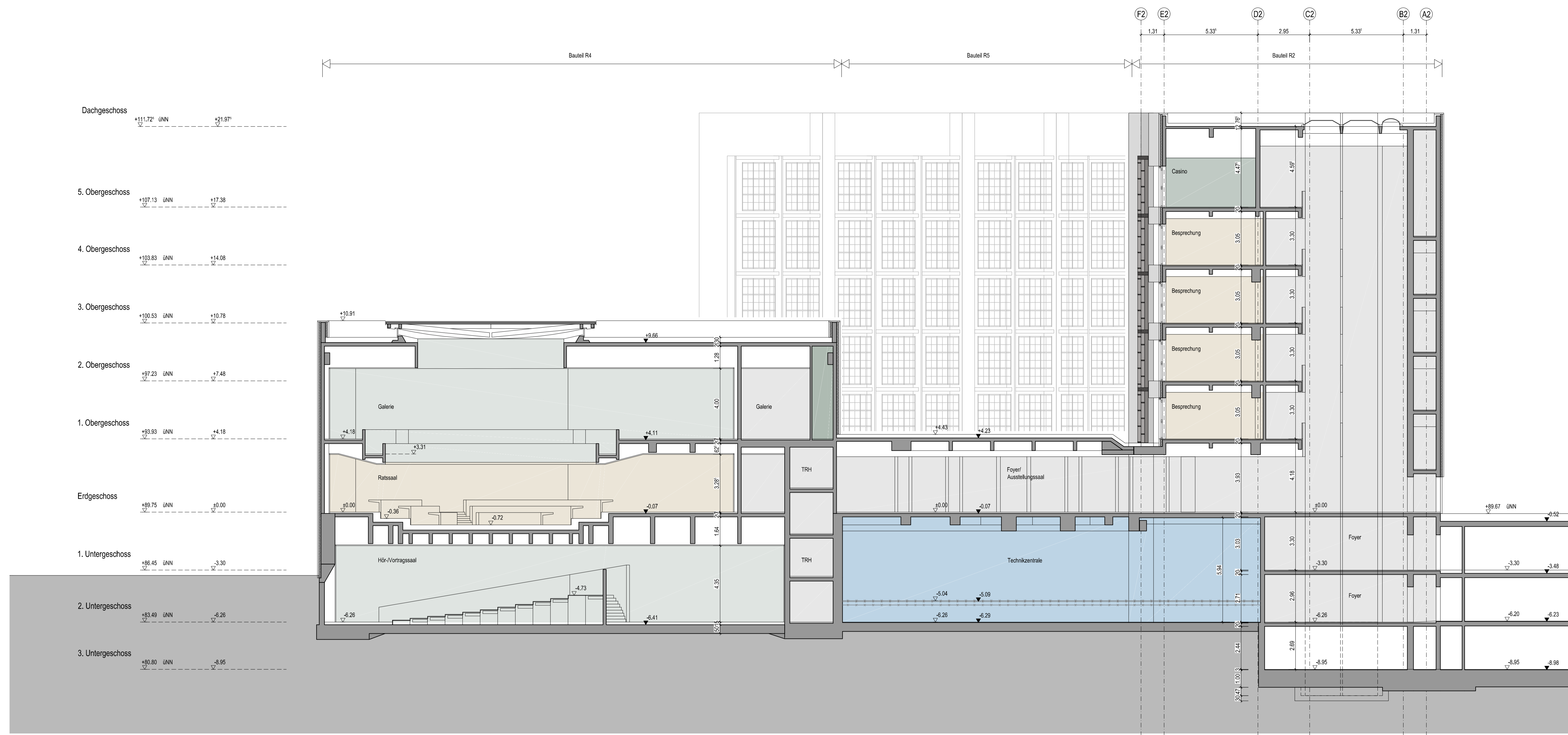
Schnitt A-A
