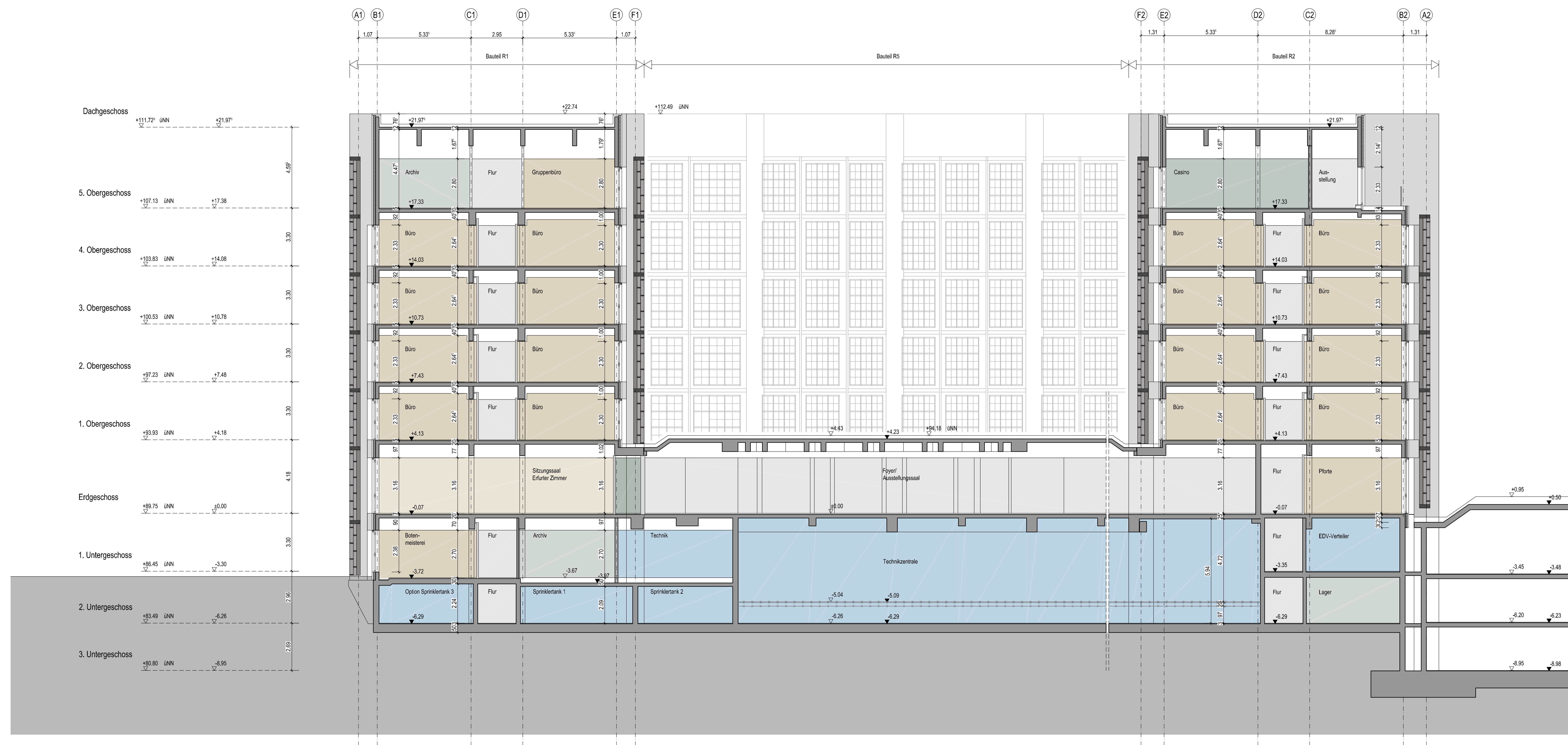
Schnitt B-B
