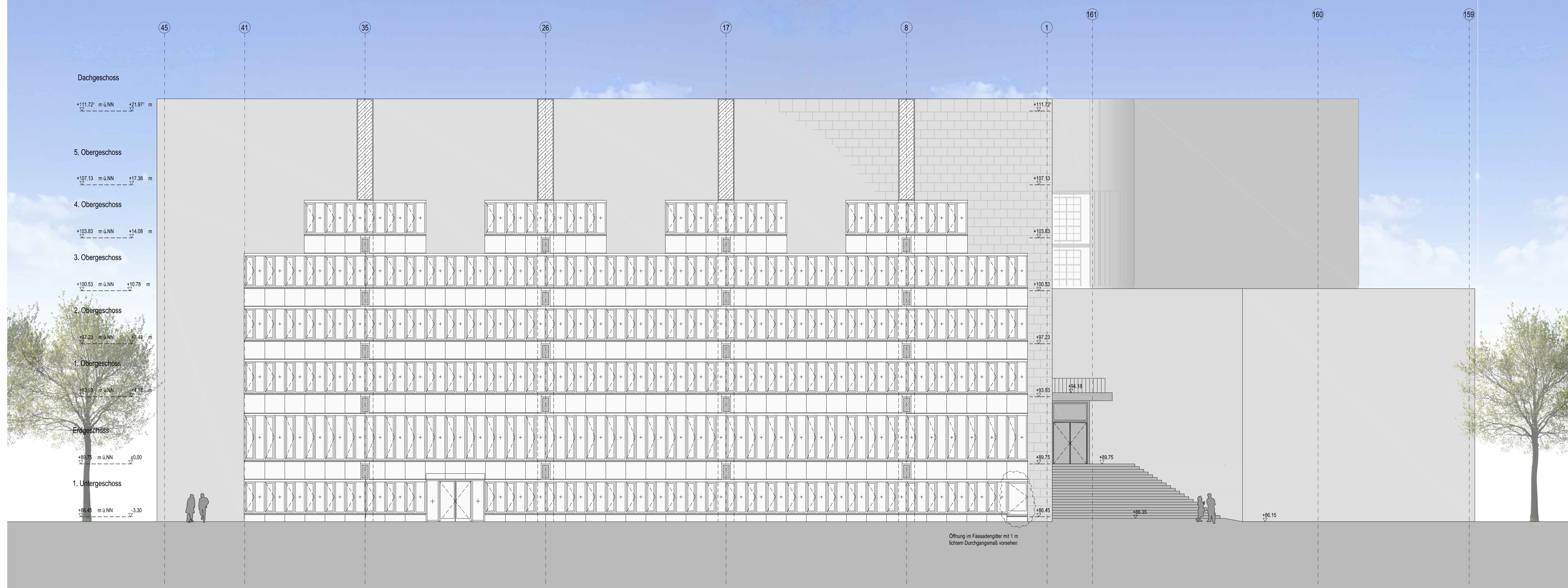
Ansicht Süd - ohne Sonnengitter
