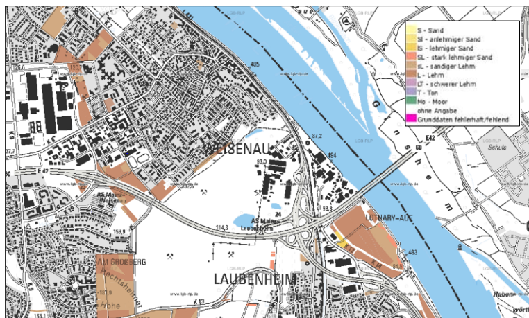
Abb. 3: Bodenarten im Bereich Mainz-Weisenau (Quelle: Landesamt für Geologie und Bergbau Rheinland-Pfalz: Bodenkarte von Rheinland Pfalz 1:10.000).
