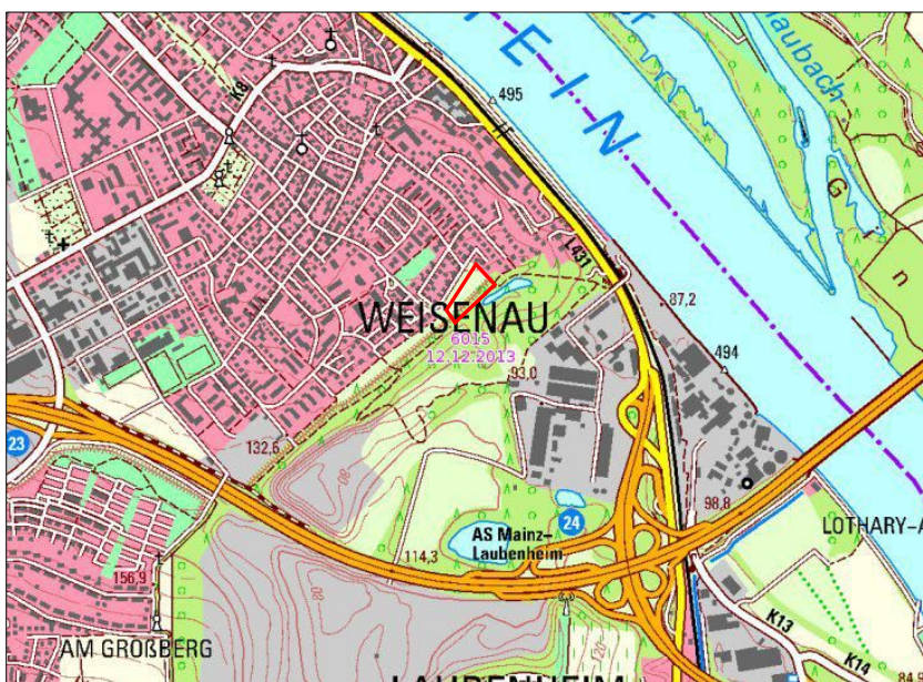
Abb. 1: Lage des Plangebiets (Ausschnitt aus der topografischen Karte DTK 25, unmaßstäblich). ( http://www.geoportal.rlp.de/portal/karten.html?WMC=2896 ).
