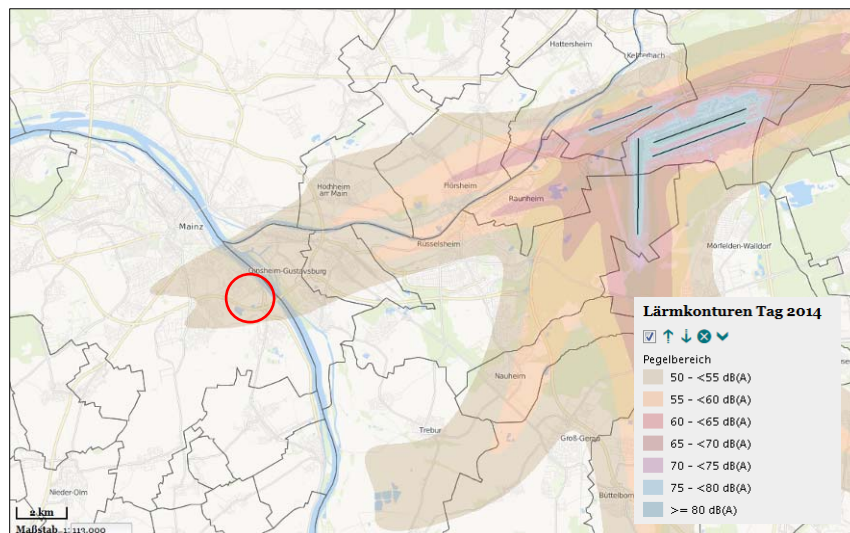
Abb. 7: „Lärmkonturen“ des Frankfurter Rhein-Main-Flughafens. 17)
