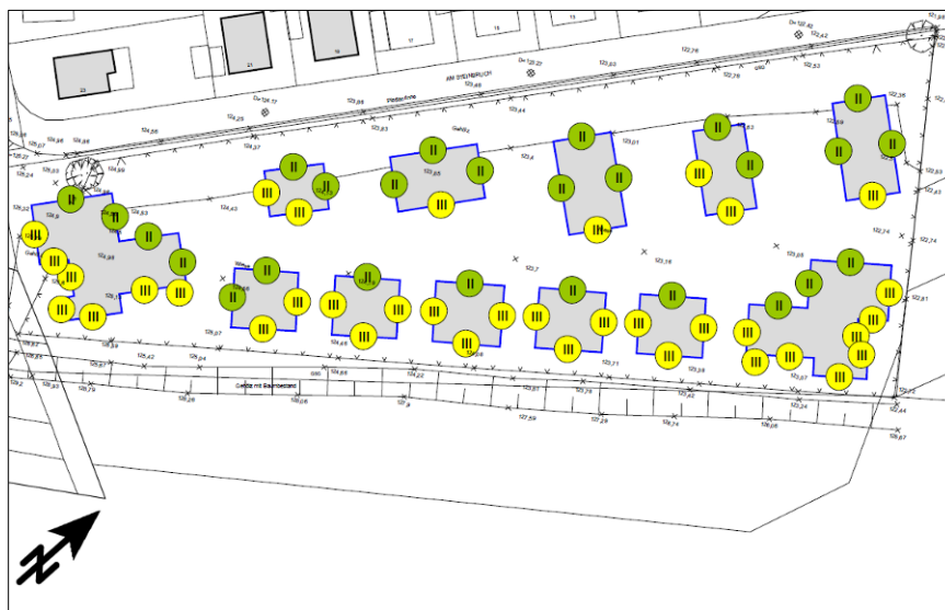
Abb. 8: Lärmpegelbereiche aufgrund der Summationswirkung verschiedener Immissionen im Plangebiet (aus FRITZ GMBH 2015).
