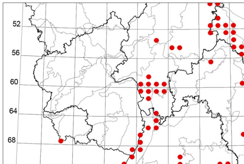
Abb. 10: Verbreitung der Mückenfeldermaus ( Pipistrellus pygmaeus ) in Rheinland-Pfalz und dem Rhein-Main-Gebiet, Stand 2006 (Quelle: BfN, http://www.ffh-anhang4.bfn.de/ffh-anhang4-mueckenfledermaus.html ). Deutlich wird die enge Bindung an das Rheintal bzw. die Mainniederung
