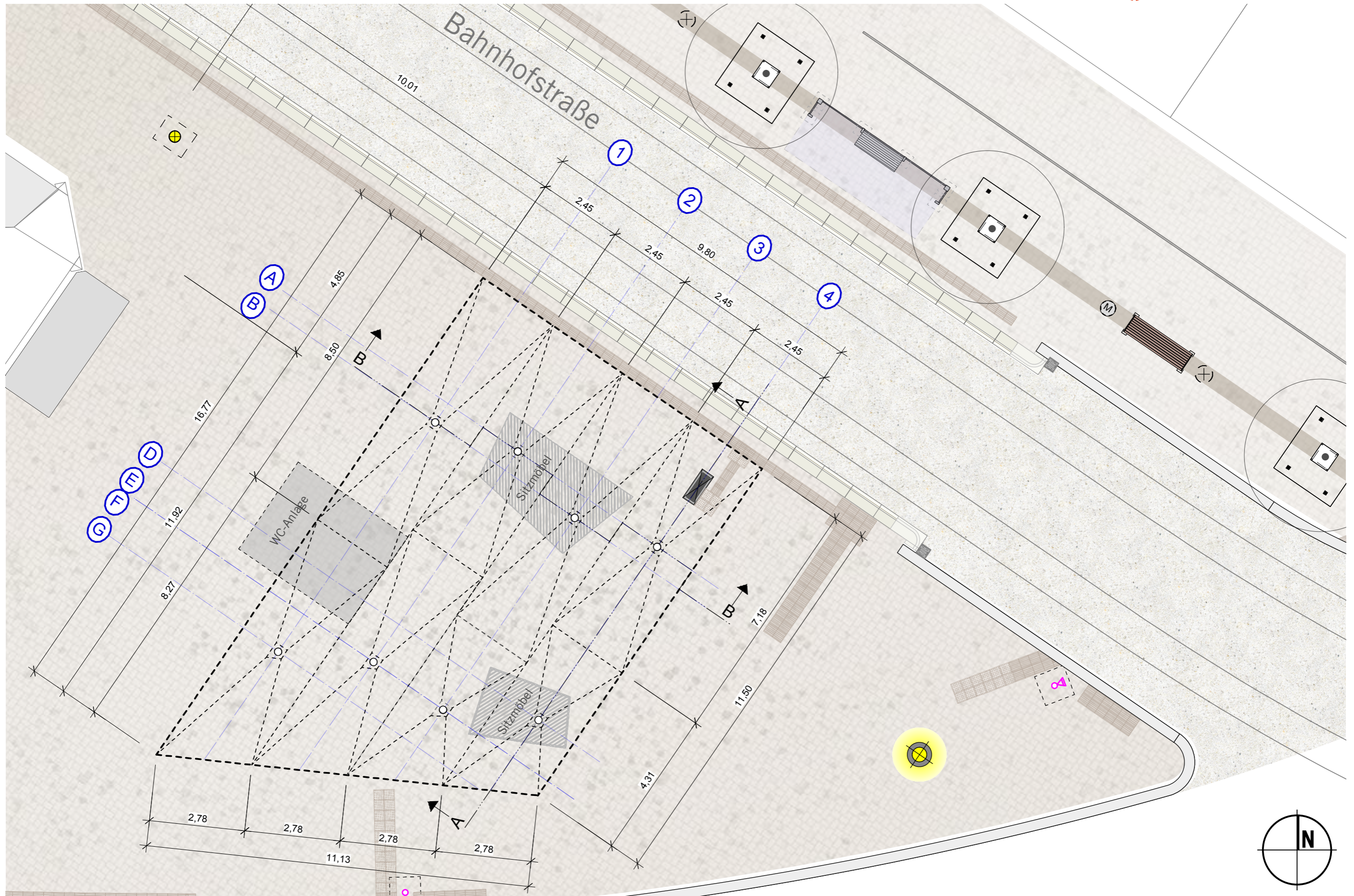
Entwurfsplanung - Flugdach mit WC-Anlage - am Münsterplatz, Mainz
