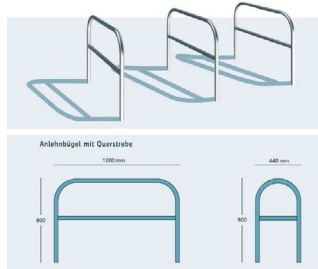
Abmessungen Citymeile Fahrradpark
