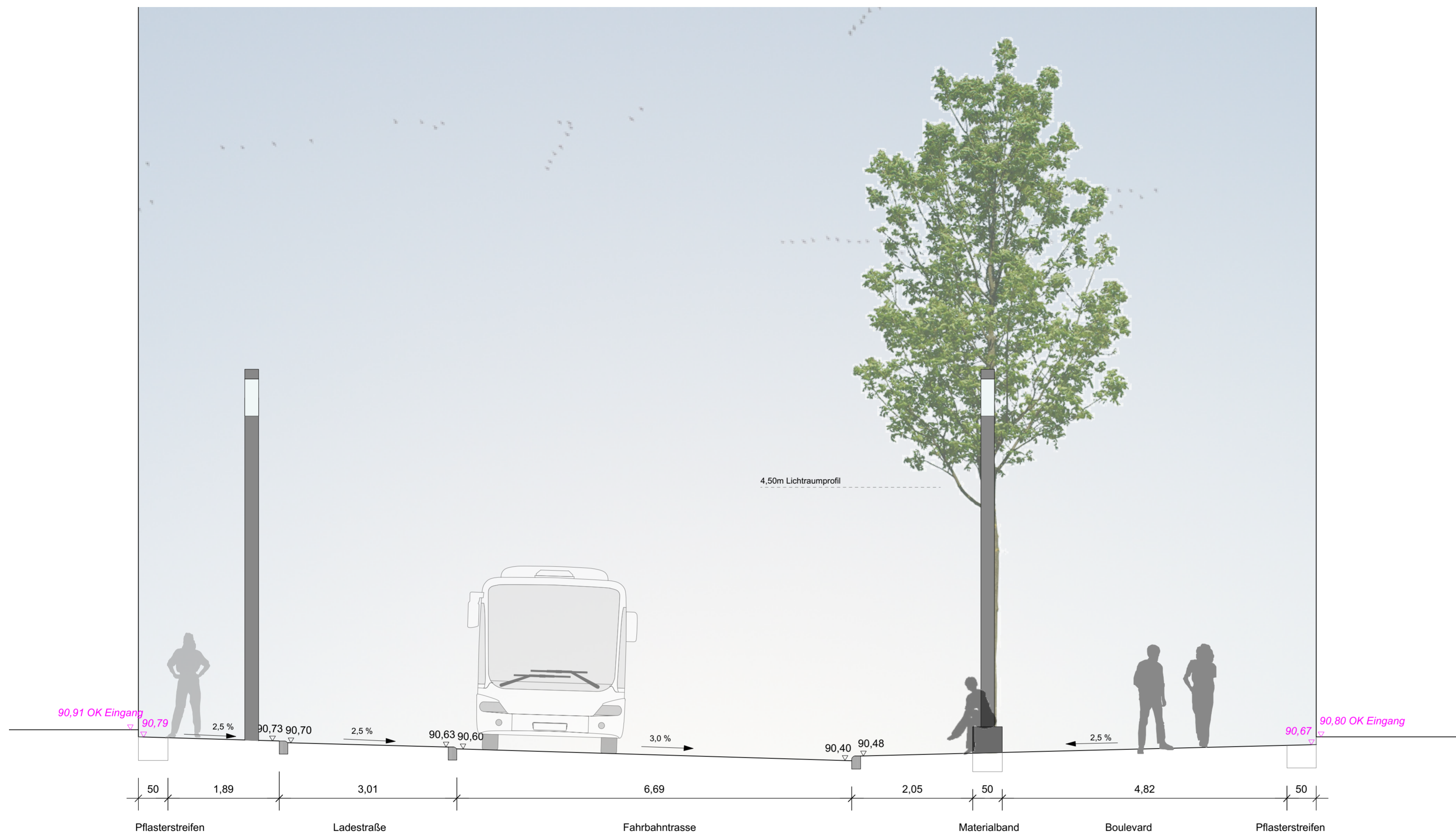
Schnitt A-A'
