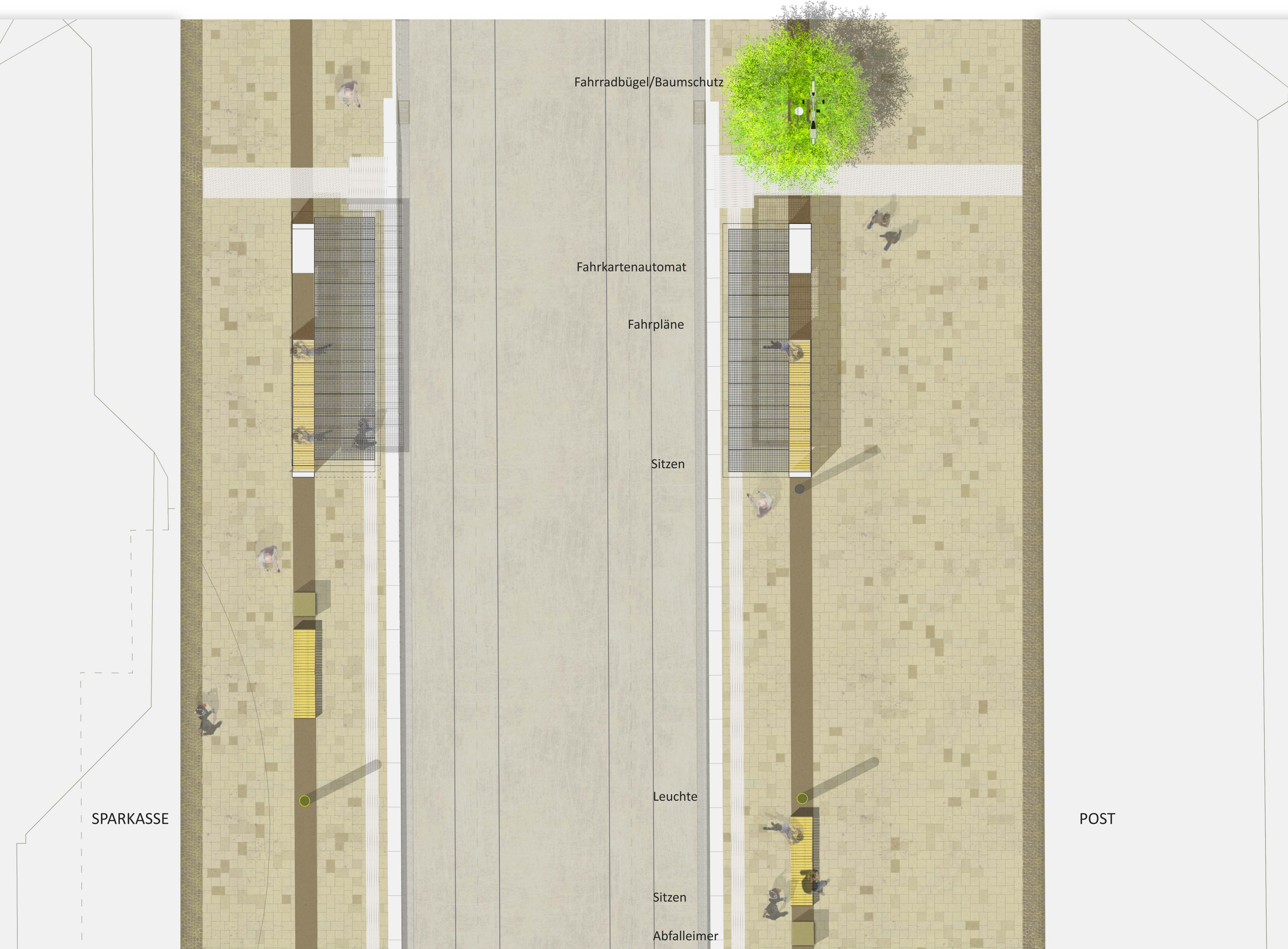
Lageplan 1:50 Vorbereich POST Gebäude VARIANTE Wettbewerb
