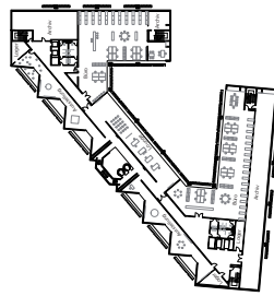
5. OG GRUNDRISS M. 1:500
