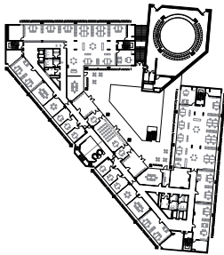
Grundriss 1.OG (jetzt 2.OG) M: 1:500
