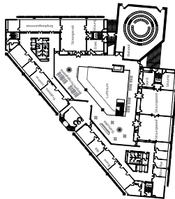
Grundriss EG (jetzt 1.OG) M. 1:500
